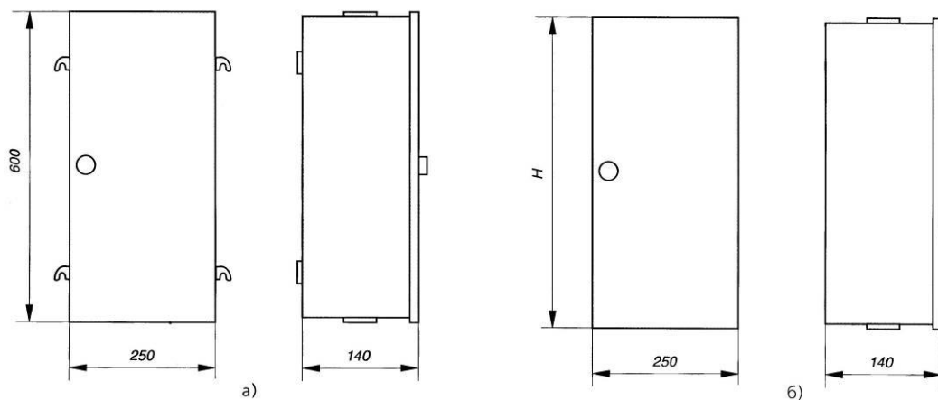
Рис № 18.4 Общий вид осветительных щитков серии ЯОУ
